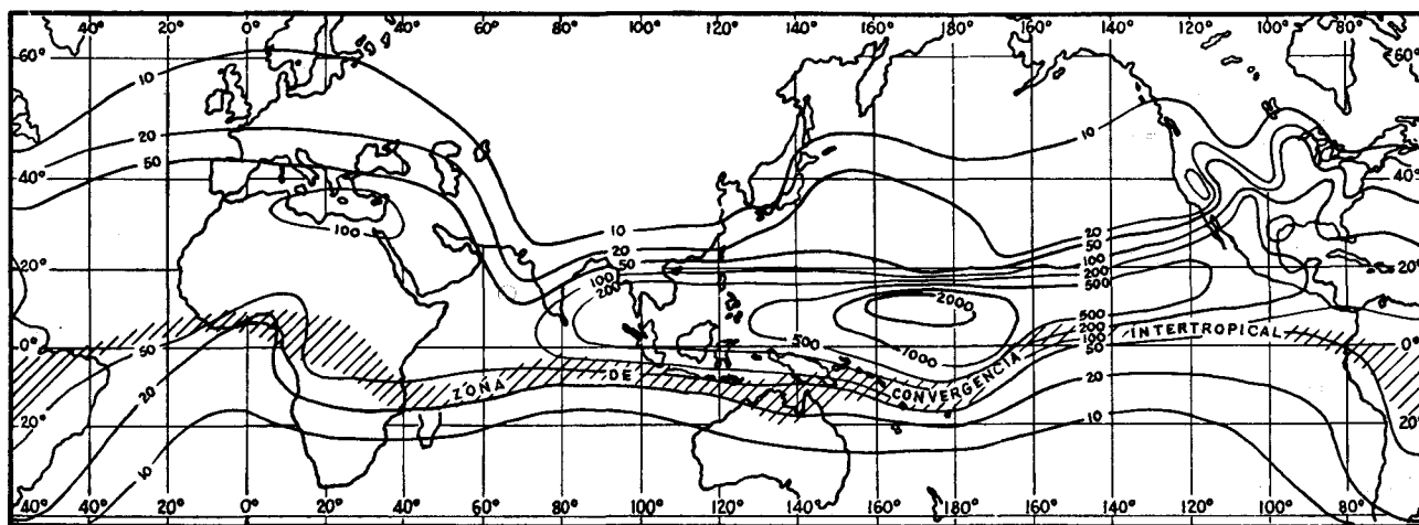
Radioactividad total de la explosión Bravo en el periodo del día 2 al día 35 después de la detonación en millicuries por 100 millas cuadradas. La zona intertropical de convergencia tiende a separar el área de los Hemisferios norte y sur cerca de la superficie de la tierra.
