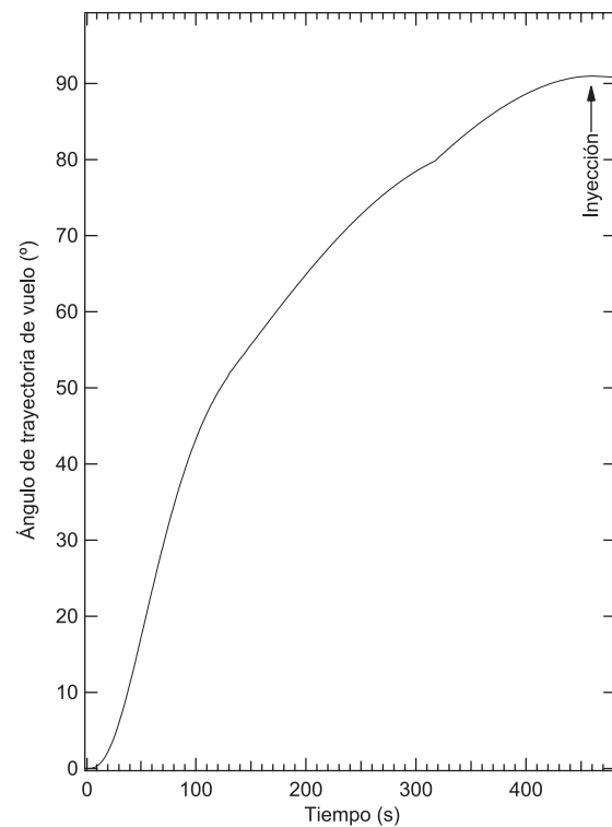
Figura 10: Comportamiento del ángulo de vuelo para un lanzamiento con azimut igual a 45^\circ .
