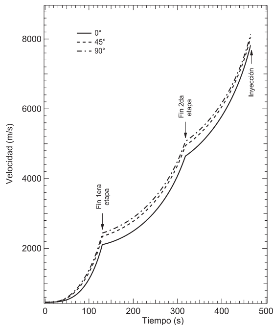
Figura 8: Perfil de velocidad del cohete con respecto al tiempo para varios valores de azimut. Se incluyeron solo los valores comprendidos a intervalos de 45° para facilitar su identificación.
