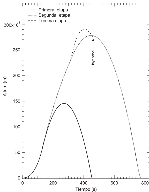
Figura 9: Comportamiento de la altura de cada una de las tres etapas para un valor de azimut de lanzamiento igual a 45^\circ .
