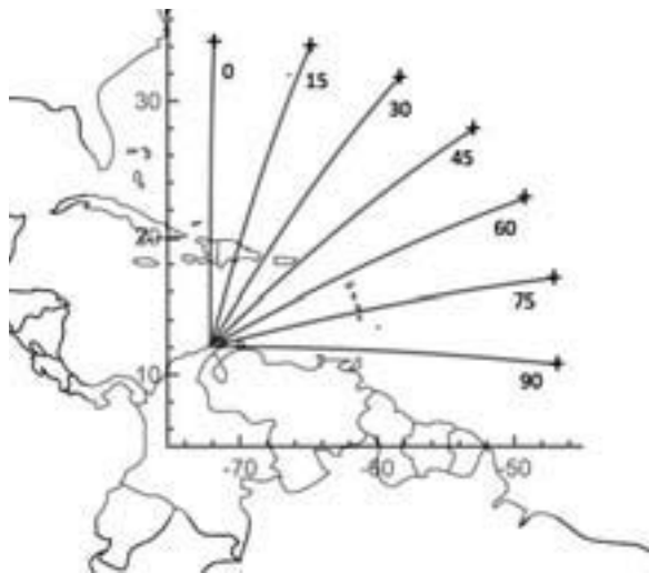
Figura 7: Trayectorias de lanzamiento del cohete con rumbos comprendidos entre 0 y 90 grados a intervalos de 15 grados. Las cruces al final de la línea señalan el lugar de impacto de la segunda etapa. Nótese que el valor de la longitud es negativo hacia el oeste.
